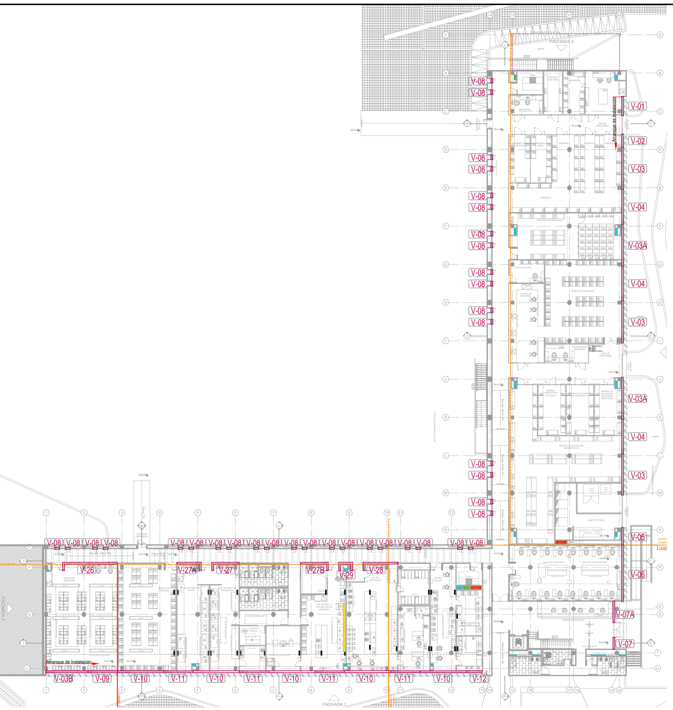
PLANTA BAJA Esc 1/250
