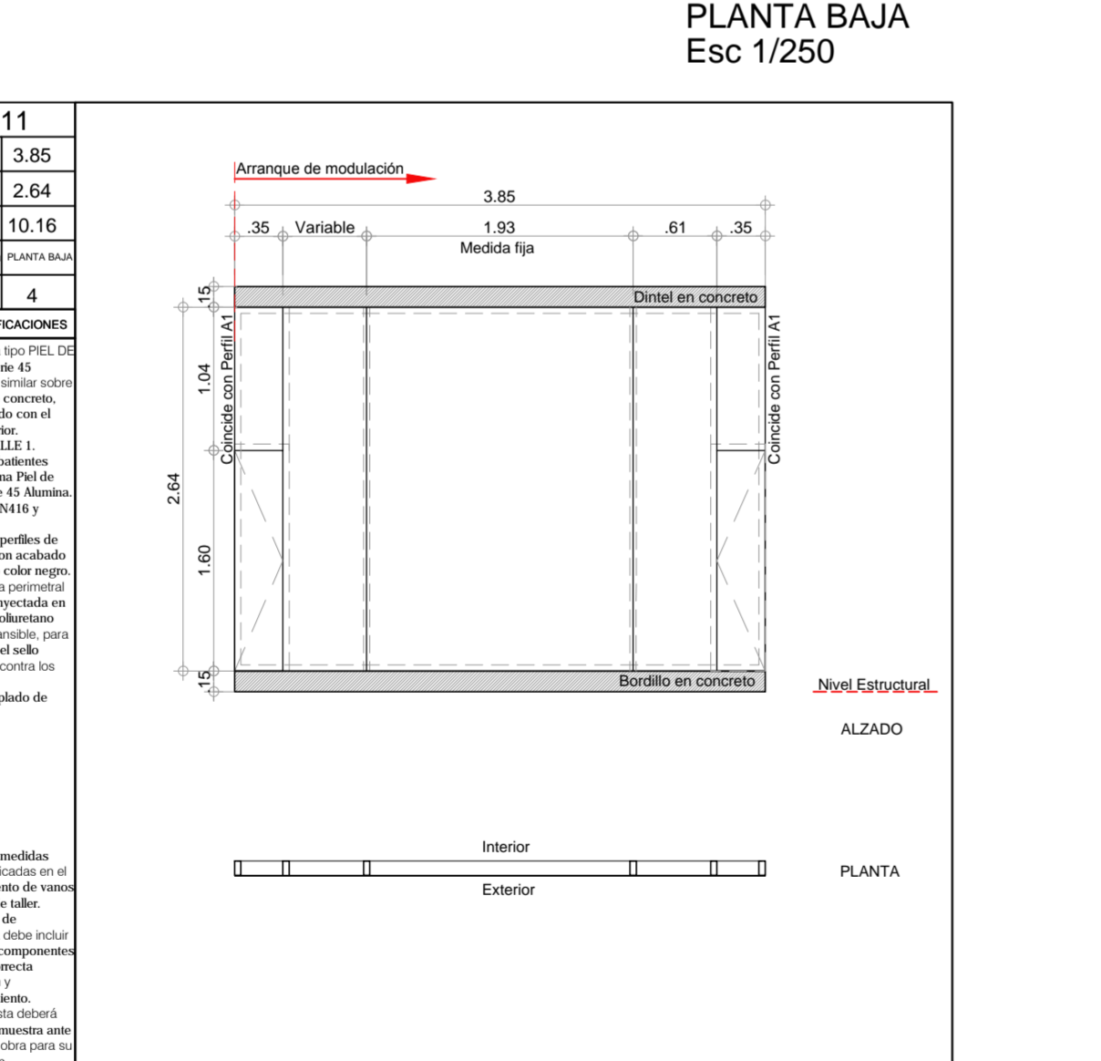
PLANTA BAJA Esc 1/250
